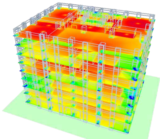
FIGUR 3. 3D-SIGNALTÄCKNINGSKARTA AV RANPLAN PROFESSIONAL
