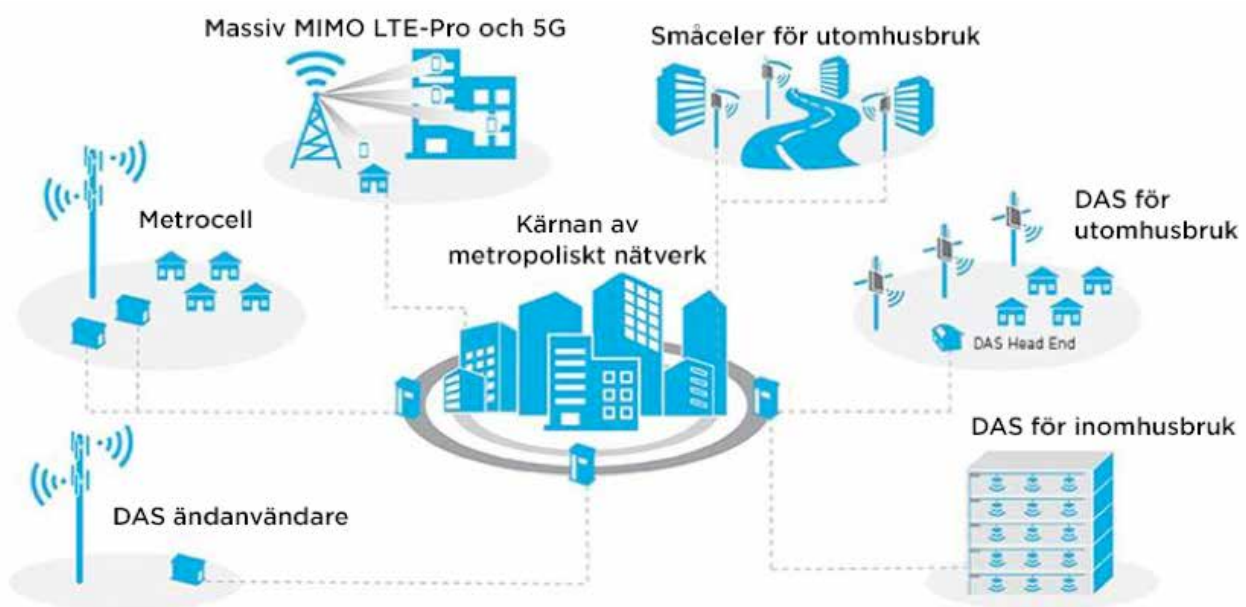
FIGUR 17. TRÅDLÖS INFRASTRUKTUR: ETT HETEROGENT NÄTVERK
