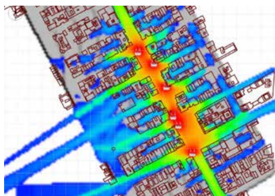
FIGUR 11. EXEMPEL PÅ TÄCKNINGSFÖRUTSEBARHET I 2D FÖR ETT WIFI-PROJEKT UTOMHUS PÅ MANHATTAN
