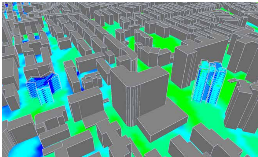
FIGUR 12. 3D-EXEMPEL PÅ EN FÖRUTSÄGELSE AV 4G TRÅDLÖST NÄTVERK INOMHUS SAMT UTOMHUS I EN TÄTBEBYGGD STADSMILJÖ
