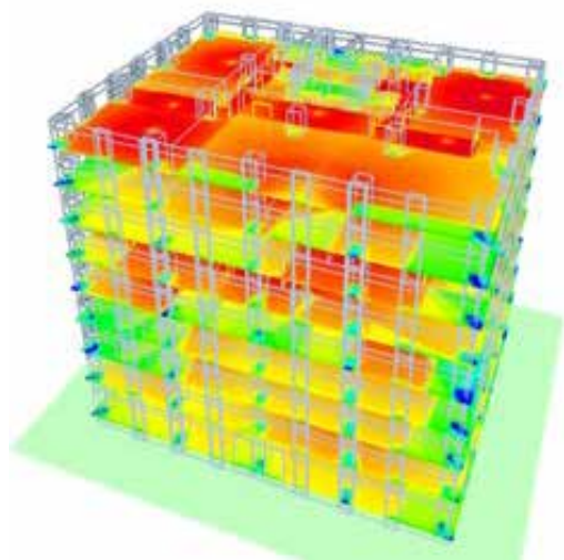
FIGUR 10. EXEMPEL PÅ TRÅDLÖS TÄCKNINGSFÖRUTSEBARHET I 3D I EN BYGGNAD
