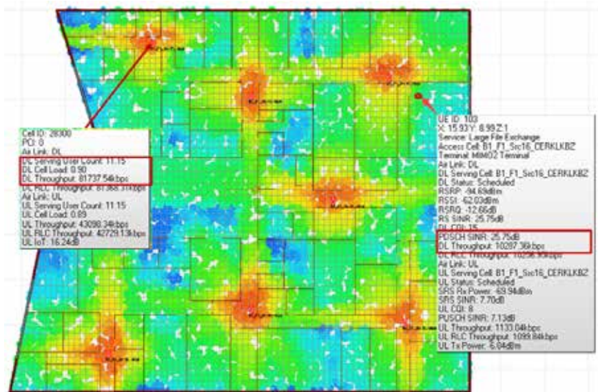
FIGUR 13. EXEMPEL PÅ ANALYS AV TÄCKNING OCH KAPACITET AV ETT 4G INOMHUSNÄTVERK.
